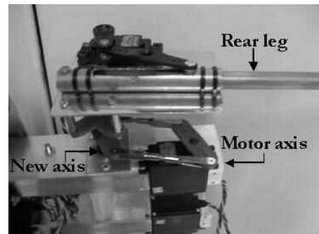
Fig. 11. Rear leg.
